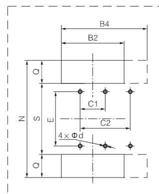
安装板的开孔尺寸(mm)
